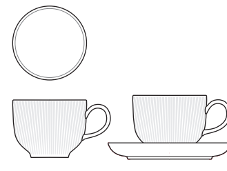
ラテカップ / 200cc latte cup w118×d90×h70
