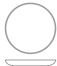
カフェプレート (ソーサー) cafe plate (saucer) Φ150×h20
